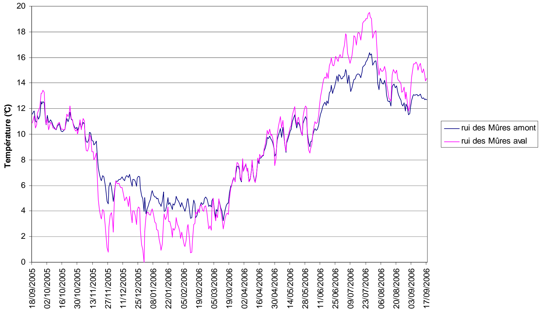
Figure 3: Courbes des températures moyennes journalières calculées sur la période du 18/09/2005 au 17/09/2006 pour les 2 stations étudiées sur le ruisseau des Mûres, affluent du Chéran.
